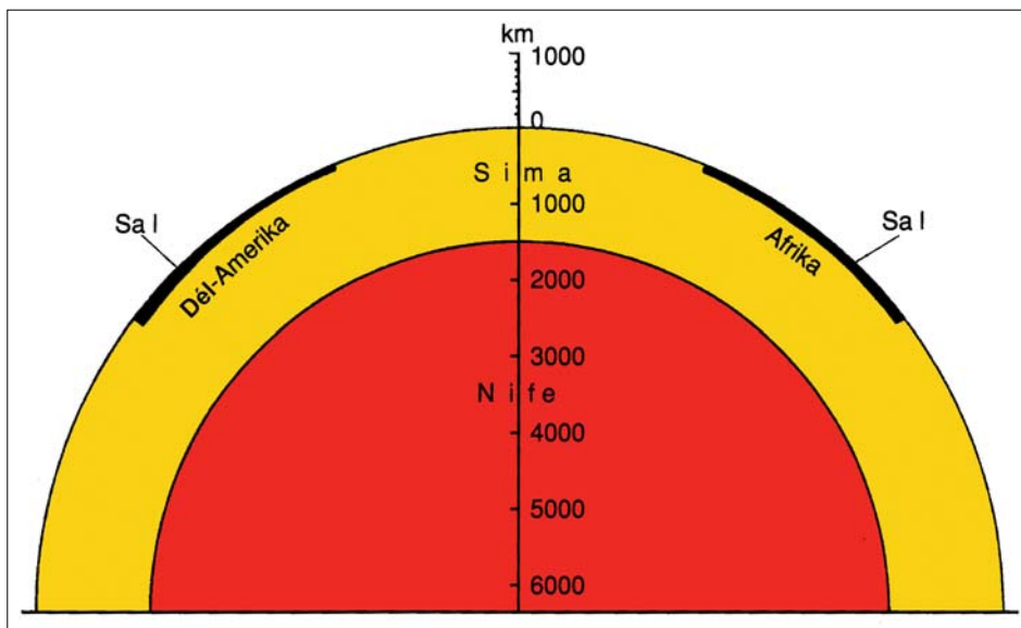
1. ábra Wegener elképzelése a Föld szerkezetéről (Wegener 1912a–b, eredeti ábra kiszínezve). A valóságosnál nagyobbak képzelt földmag (Nife) felett húzódó bazaltos összetételű és viszkózus „Sima” földhéjban (földköpenyben) úsznak a kontinensek (Sal).
